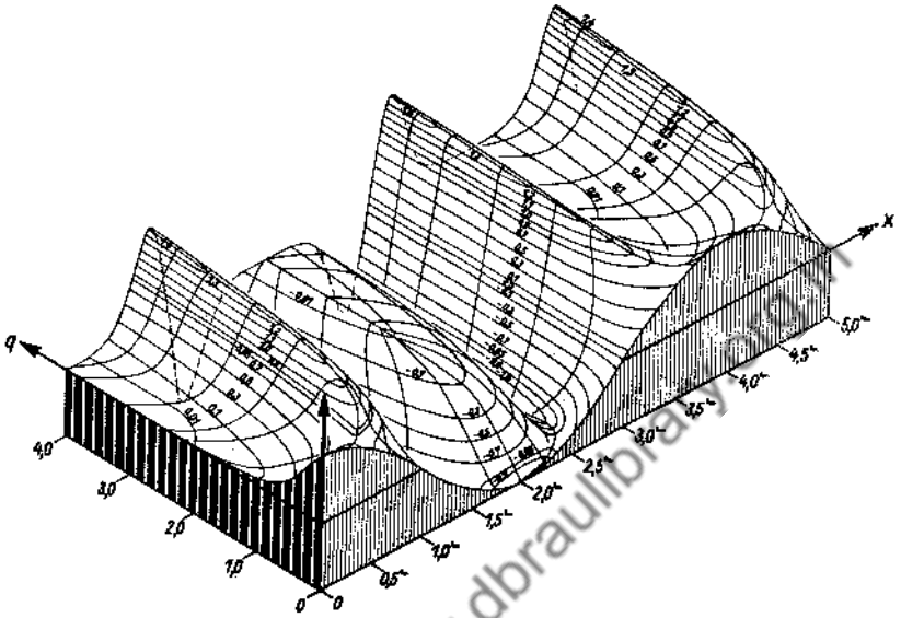
Fig. 170. ce_1(x, q) .
