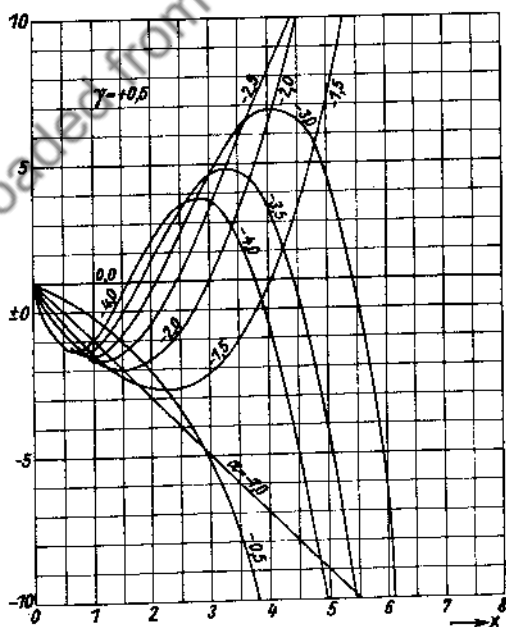
Fig. 154. M(\alpha, +0,5, x) .
