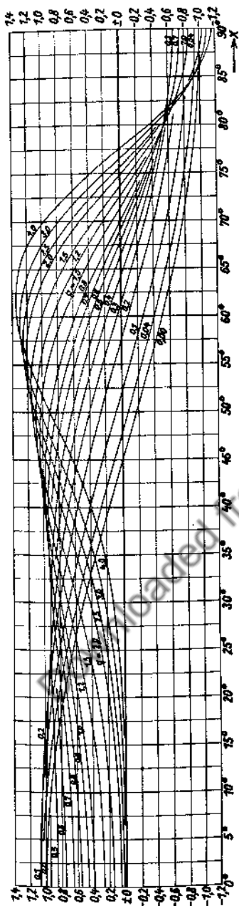
Fig. 176. ce_2(x, q) .
