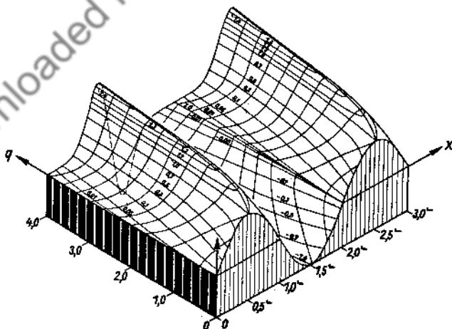
Fig. 175. se_2(x, q) .
