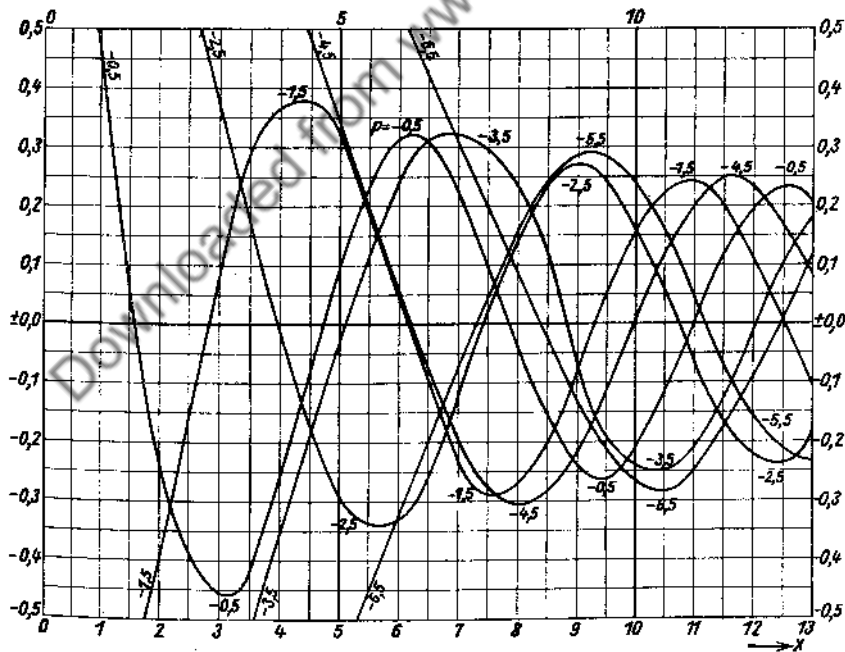
Fig. 86. J_{-n-0.5}(x) .
