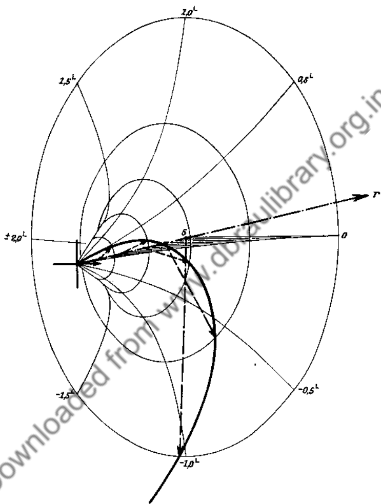
Fig. 141. Die Pfeile b i^{\beta} = J_1(r \sqrt{i}) senkrecht von der r -Achse ausgehend. (vgl. S. 262.) Beispiel: Magnetische Wechselfeldstärke im Runddraht in verschiedenen Abständen von der Drahtachse.
