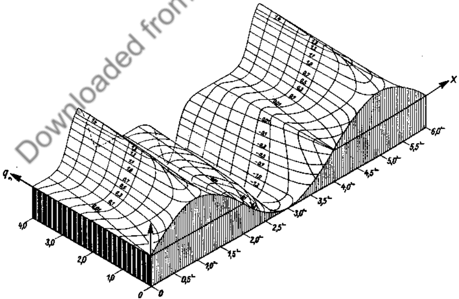
Fig. 171. se_1(x, q) .
