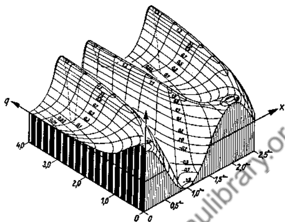
Fig. 174. ce_2(x, q) .
